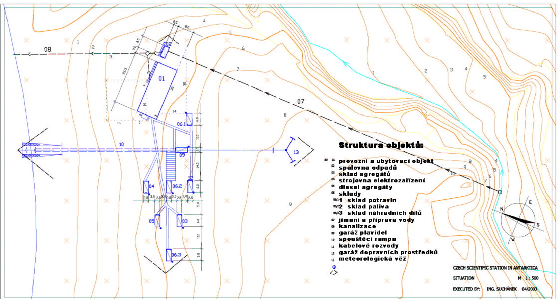
Obt. 4 Plánovaná struktura objektů české vědecké stanice v Antarktidě (zdroj: http://www.national-geographic.cz )
